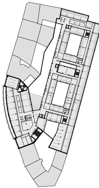
Regelgeschoss
